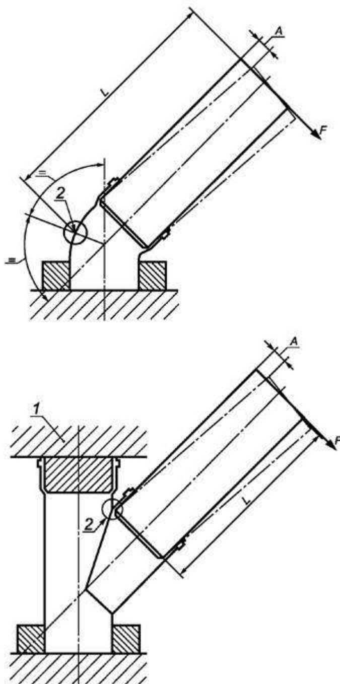
1 - фиксирующие элементы; 2 - зона возможного разрушения
