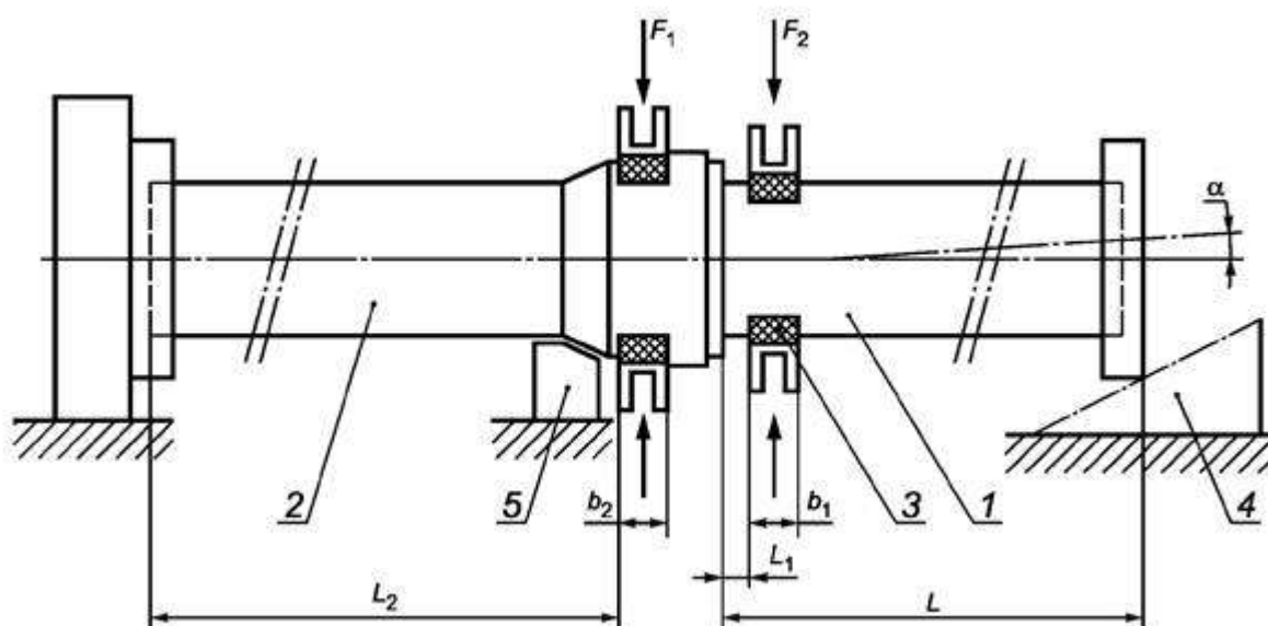
1 - труба; 2 - труба или фланцевая часть с раструбом L_2 \geq 1000 мм; 3 - зажимы; 4 - регулируемая опора для создания осевого смещения; 5 - фиксатор раструба
